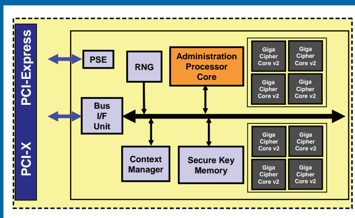
NITROX PX CN15XX - Block Diagram
